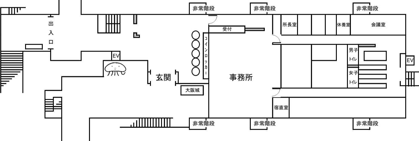
【 宿泊管理棟 地下 】
